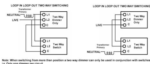
Wiring
